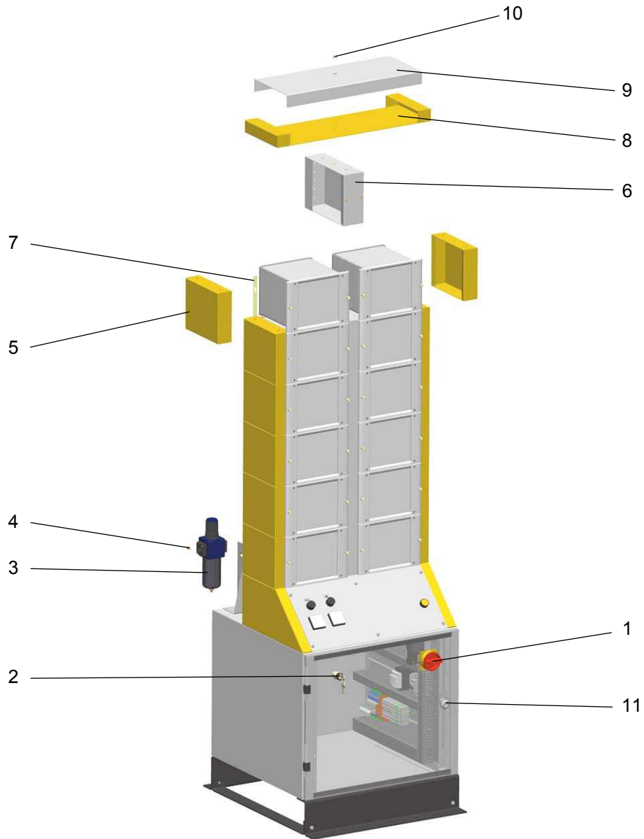
OptiFlex A1-sokkelkast - Onderdelen
