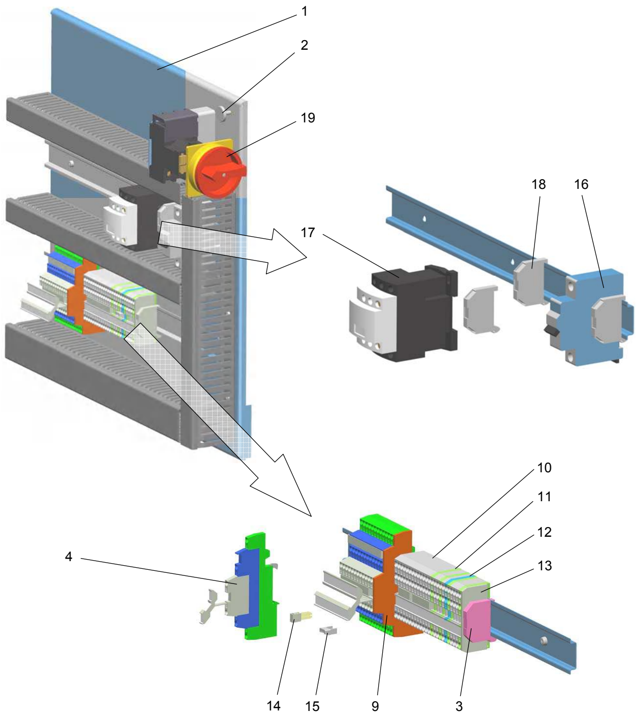
OptiFlex A1 - Inbouwplaat
