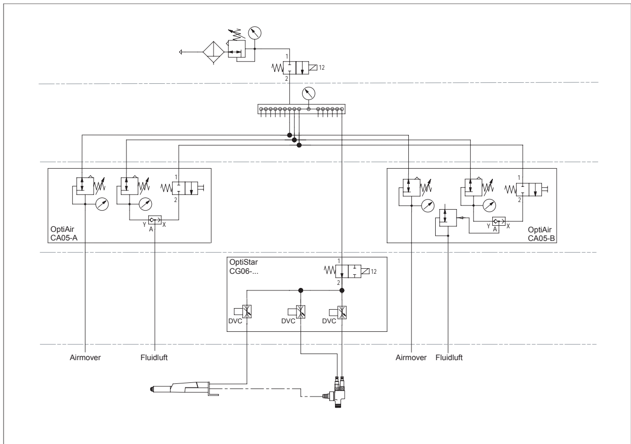
Besturingssysteem OptiFlex A1 - Pneumatisch schema
